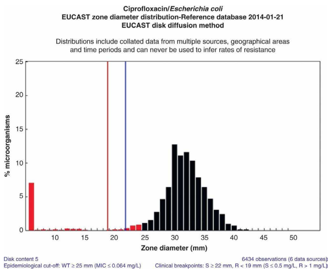
Figura 3. Distribuzione del diametro della zona di inibizione di E. coli in seguito al passaggio da “MIC” a “Diffusione su disco”.
