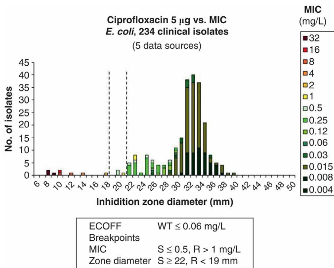
Figura 4. **Relazione tra le MIC di E. coli ciprofloxacina e i diametri delle zone di inibizione utilizzati da EUCAST per determinare la correlazione tra le MIC e i diametri delle aree e per determinare i breakpoint dei diametri delle aree. I dati sono disponibili all’indirizzo: http://www.eucast.org/antimicrobial_susceptibility_testing/calibration_and_validation/ .
