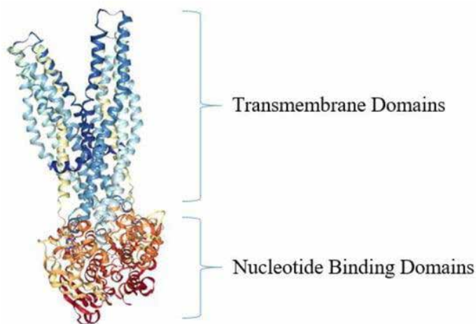
Figura 5. Struttura cristallina della pompa di efflusso ABC batterica di S. aureus . La porzione superiore del trasportatore ABC Sav1866 è rappresentata in blu e azzurro e rappresenta i due TMD (talvolta chiamati domini di membrana, MSD) della proteina, mentre i colori arancione e rosso raffigurano i due NBD [104]. Il modello di struttura è stato generato utilizzando NGL Viewer [106] delle voci 2HYD e 2ONJ del PDB [107], come riportato [104,108].
