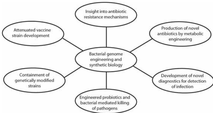
Figura 3. L'uso di strumenti di SB e di ingegneria genomica per contrastare le infezioni batteriche. Immagine a grandezza naturale
