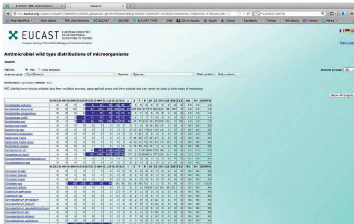
Figura 1. **Distribuzioni delle MIC di ciprofloxacina dell'EUCAST dal sito web dell'EUCAST.
