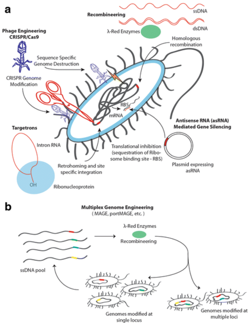
Figura 1. a) Schema degli strumenti di ingegneria genomica sviluppati in E. coli ed estesi a molti altri ospiti batterici b) Multiplexed Automated Genomic Engineering (MAGE) per modificare i batteri in più loci genomici. Immagine a grandezza naturale
