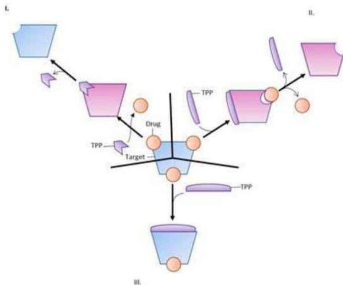
Figura 4. Tipi di meccanismi di protezione del bersaglio antimicrobico. (I) La proteina di protezione del bersaglio (TPP) riguarda direttamente l'agente antimicrobico dal suo sito attivo sul bersaglio, impedendo l'azione antimicrobica. (II) La proteina di protezione del bersaglio lega un sito allosterico del bersaglio, che induce un cambiamento di conformazione e la dissociazione dell'agente antimicrobico dal sito del bersaglio. (III) La proteina di protezione del bersaglio induce un cambiamento conformazionale globale per ristabilire la funzione del bersaglio nonostante la formazione di un complesso bersaglio-farmaco [84]. Questa figura è stata gentilmente fornita da Ann F. Varela.
